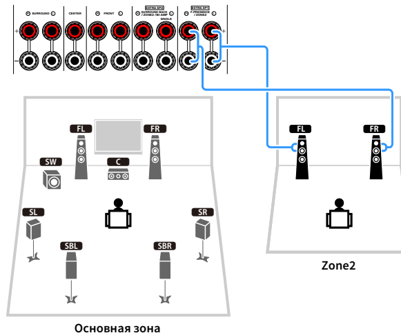
Аппарат (вид сзади)
