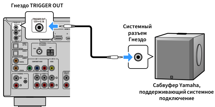
Аппарат (вид сзади)
