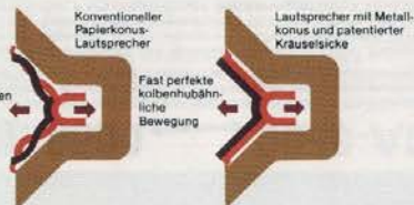
Lautsprechervergleich Papierkonus: Metallkonus/Kräuselsicke
