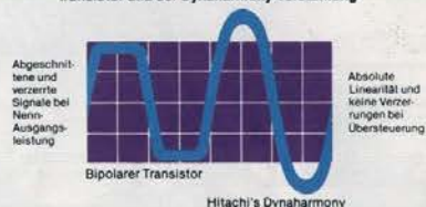
Graphische Darstellung: Simulierte Oszillogramme aus dem Hitachi-Laboratorium in Toyokawa
