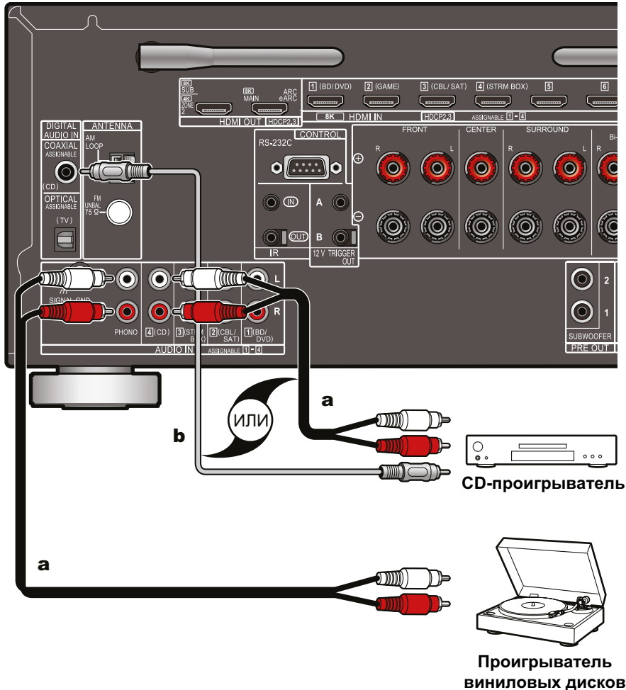
a Аналоговый аудиокабель b Цифровой коаксиальный кабель
