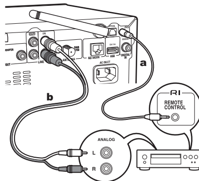
a RI-Kabel, b Analoges Audiokabel
