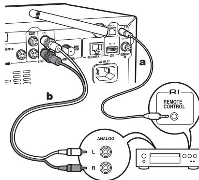
a Cavo RI, b Cavo audio analogico
