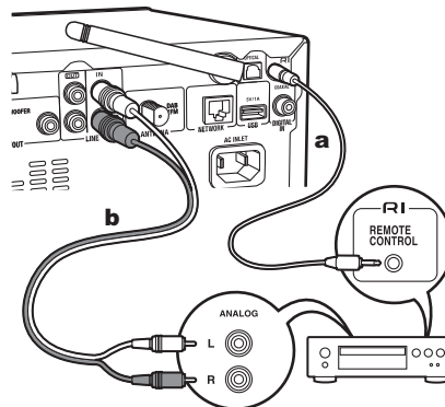
a RI-kabel, b Analoge audiokabel
