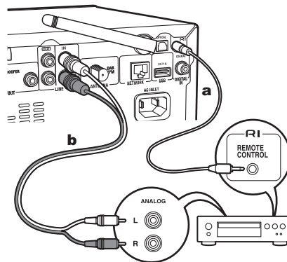
a Câble RI, b Câble audio analogique
