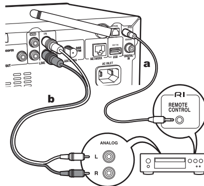
a Cable RI, b Cable de audio analógico
