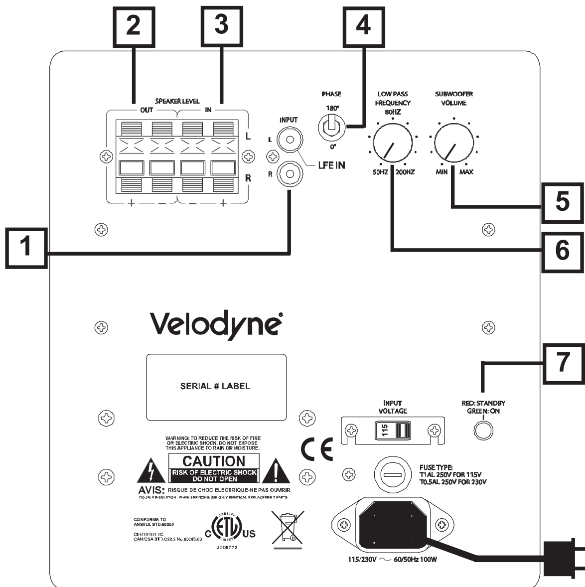
Рисунок 1. Органы управления и соединительные разъемы на задней панели сабвуфера Impact
