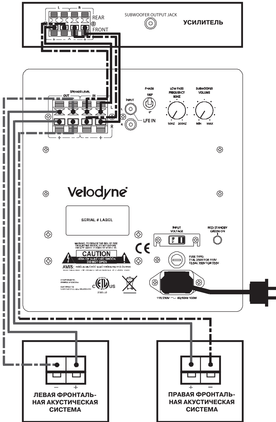
Рисунок 26. Схема подключения сабвуфера с применением соединений уровня громкоговорителей
