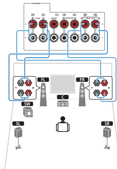
Аппарат (вид сзади)
