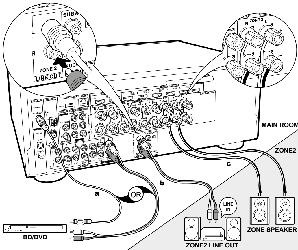
a Цифровой оптический кабель или цифровой коаксиальный кабель, b Аналоговый аудио кабель, c Колоночный кабель
